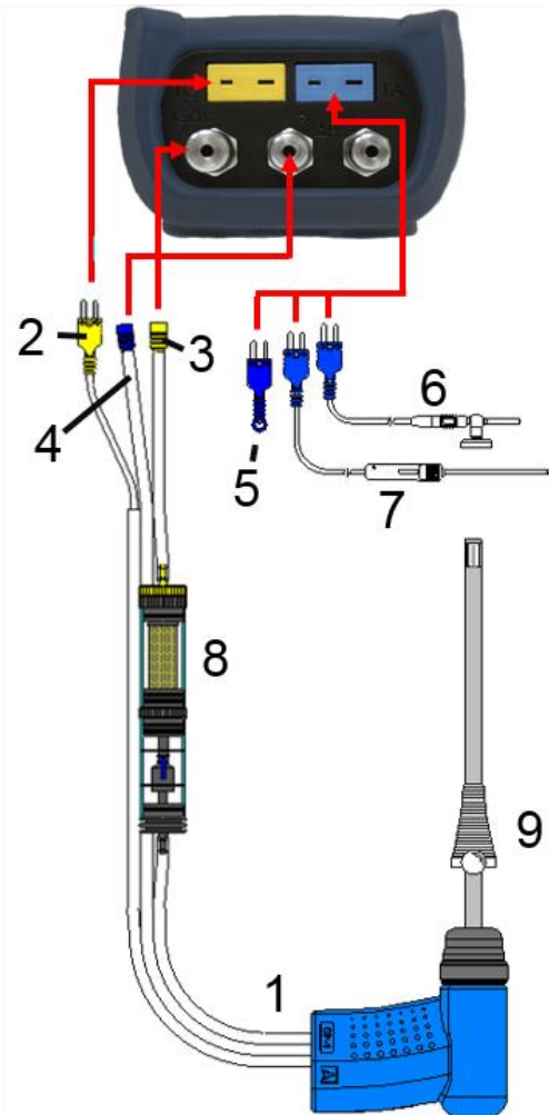
Bild 1: Anschlussschema (Sensorseite)
