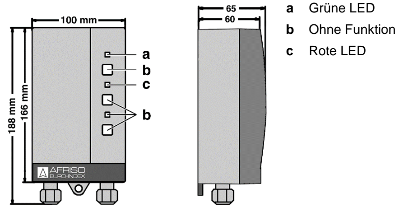
Bild 4: EMS 220
