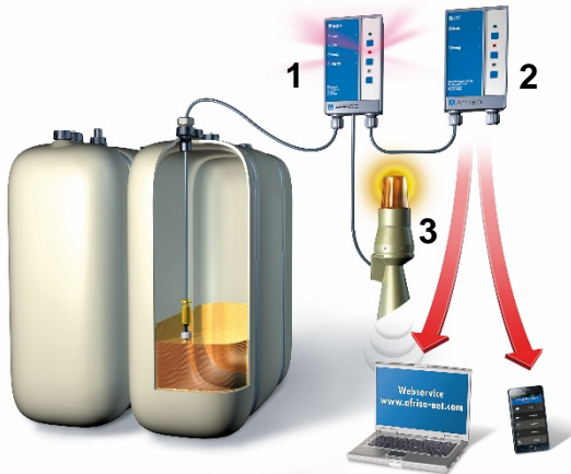
Bild 2: Anwendungsbeispiel EMS 220
