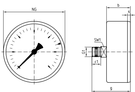
HZ 80 – Anschluss axial, zentrisch
